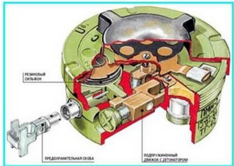
Рис.2 Разрез мины ПМН-2
